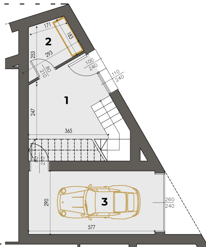
PIANTA PIANO TERRA - 1:100
